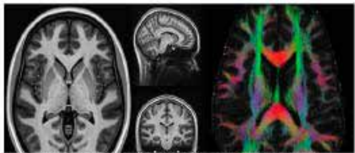
IRM structurale cérébrale de très haute résolution à ultra-haut champ (7T) (CRMBM-CEMEREM, UMR AMU-CNRS 7339 & APHM)
