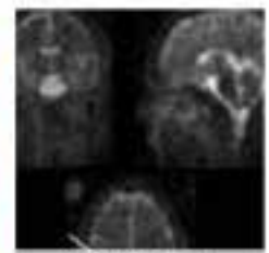
IRM Cérébrale du sodium (CRMBM)
