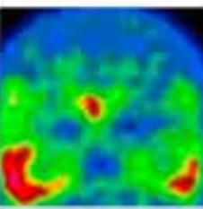
Imagerie de la protéine Tau Imagerie PET (CERIMED)
