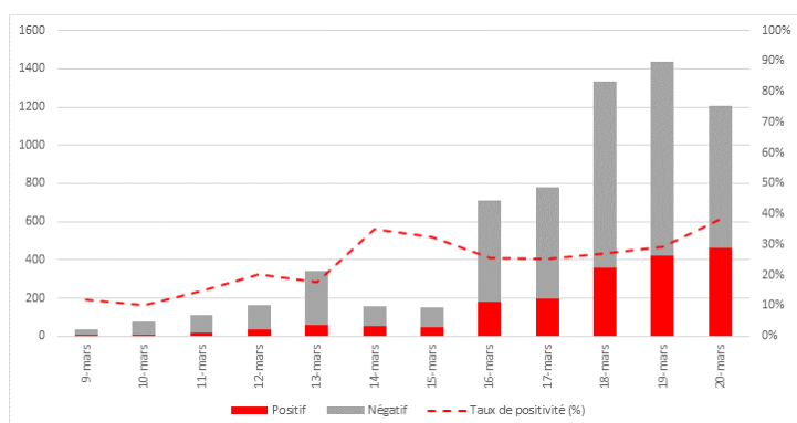
Figure 5. Nombre de tests réalisés par les laboratoires de ville, nombre de tests positifs et taux de positivité pour le SARS-CoV-2 par jour, France, du 24 février au 24 mars 2020 (N total = 6500 tests, n positifs = 1845 tests) (source : Surveillance 3 labo)
